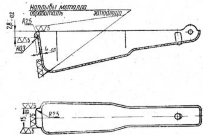
Рис. 57. Крышка магазина
