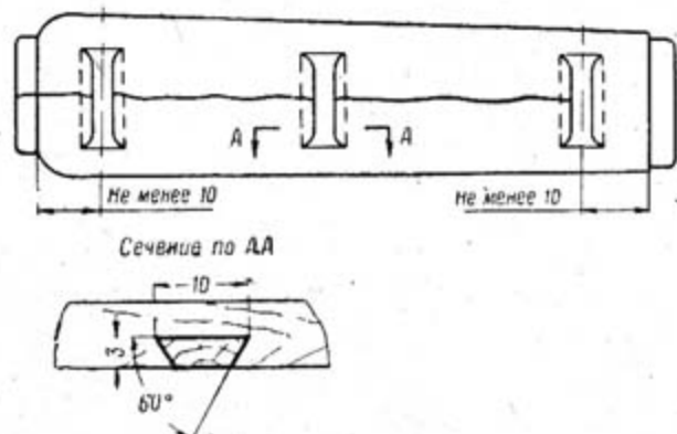
Рис. 55. Ствольная накладка
