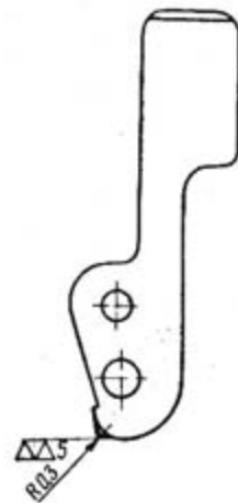
Рис. 16. Курок
