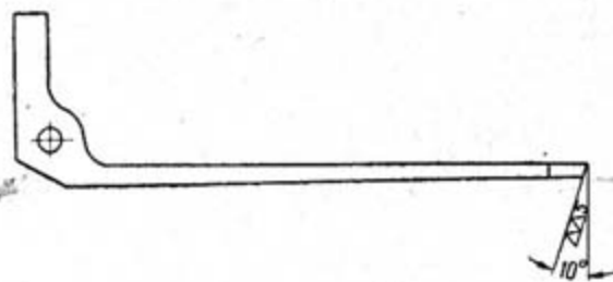
Рис. 21. Спусковой рычаг
