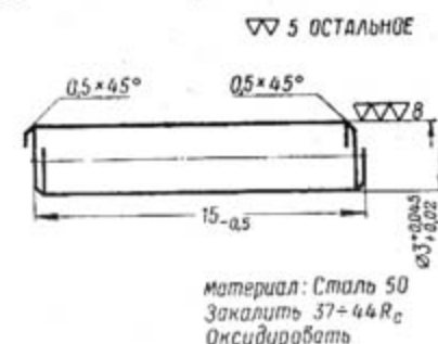
Рис. 1. Штифт
