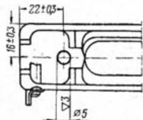
Рис. 23. Ствольная коробка
