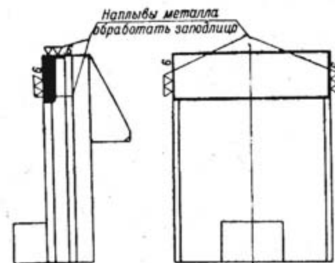
Рис. 64. Останов затвора
