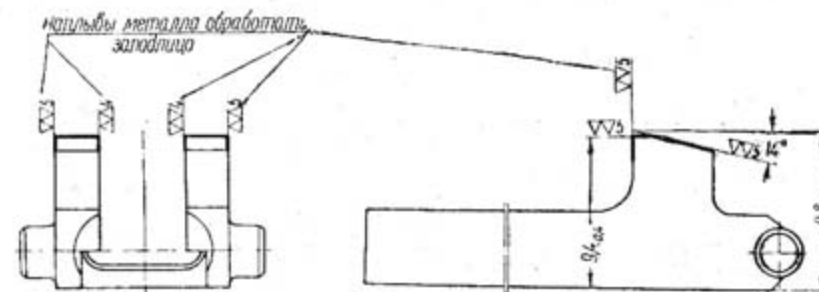
Рис. 17. Разобщитель
