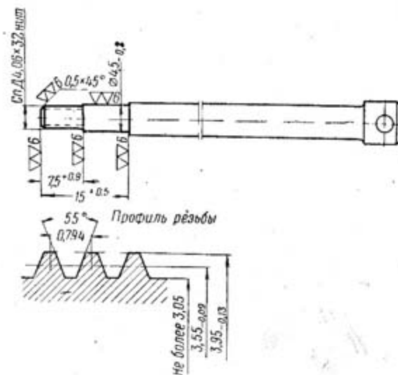
Рис. 70. Шомпол
