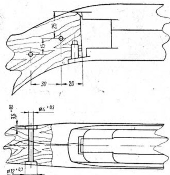
Рис. 38. Обработка отверстия для шпилек в шейке ложи
