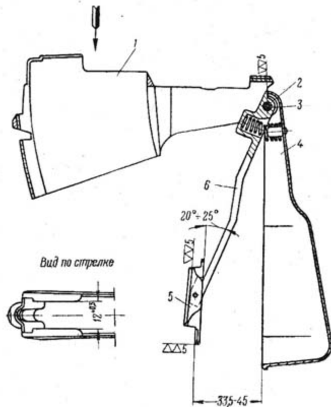
Рис. 59. Магазин:
