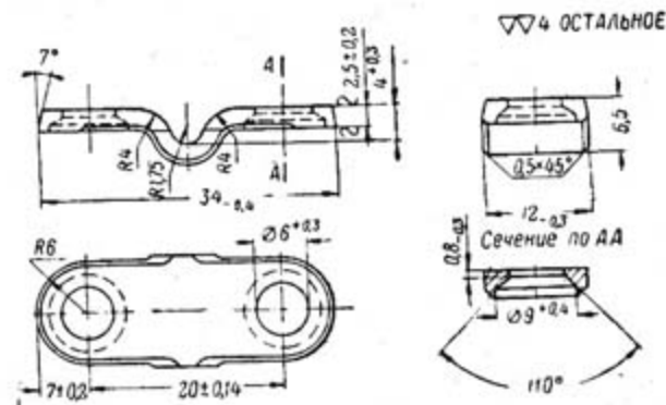
Рис. 47. Основание антабки
