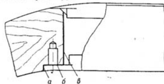
Рис. 72. Подчистка ложки
