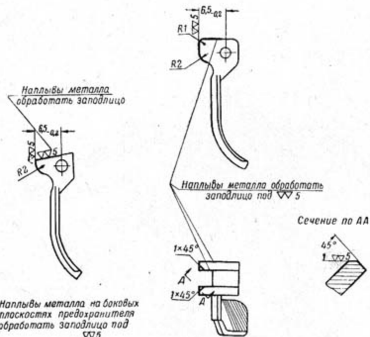
Рис. 25. Предохранитель карабинов последних годов изготовления
