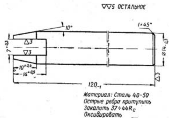
Рис. 74. Оправка для правки трубки ствола
