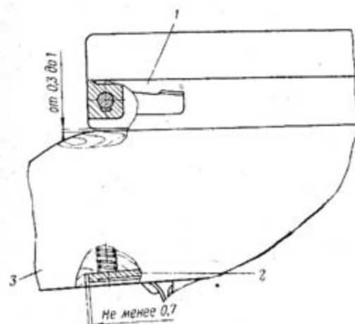
Рис. 73. Сборка ложки со ствольной коробкой и ударно-спусковым механизмом: 1 — ствольная коробка; 2 — спусковая скоба; 3 — ложка
