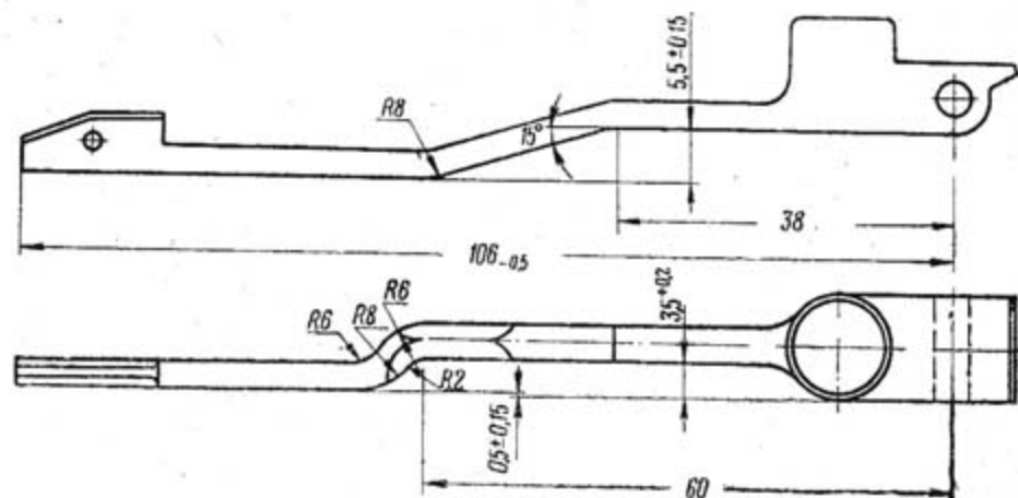
Рис. 58. Рычаг подавателя
