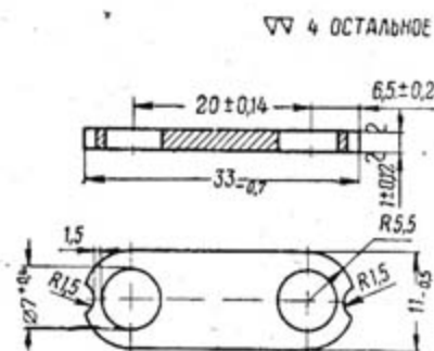
Рис. 49. Пластинка антабки
