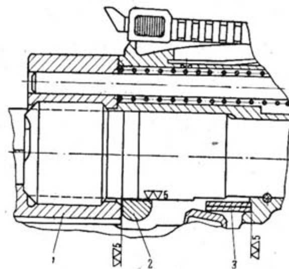
Рис. 42. Пригонка нагеля и магазина: 1 — ствольная коробка; 2 — нагель; 3 — магазин
