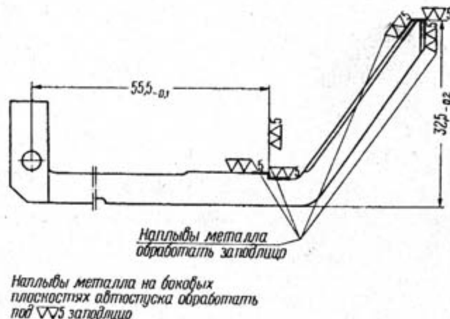
Рис. 20. Автоспуск
