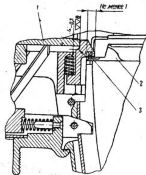
Рис. 60. Пригонка останова затвора: 1 — осто́в затвора; 2 — подаватель; 3 — останок затвора
