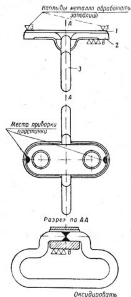
Рис. 50. Антабка ложи: 1 — пластинка антабки; 2 — основание антабки; 3 — кольцо антабки
