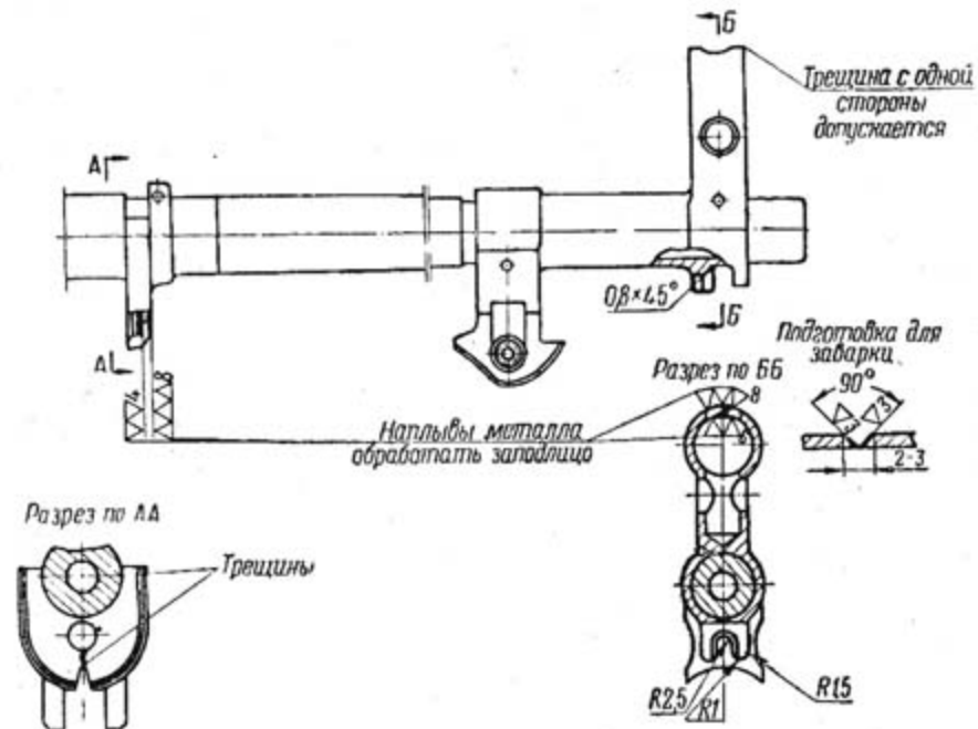
Рис. 9. Ствол
