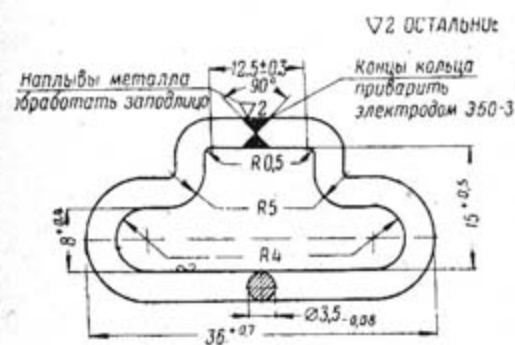
Рис. 47. Основание антабки
