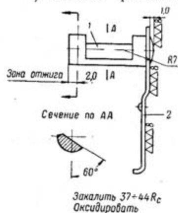
Рис. 54. Чека накладки:
