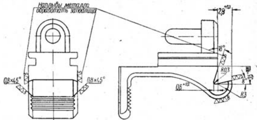
Рис. 56. Защелка крышки магазина
