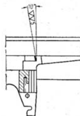
Рис. 13. Зачистка отражающего выступа ствольной коробки
