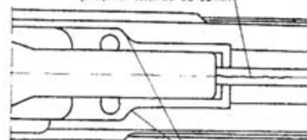
Рис. 40. Постановка вклеек с обработкой их концов под углом 90°
