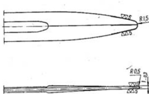
Рис. 68. Штык клинковый
