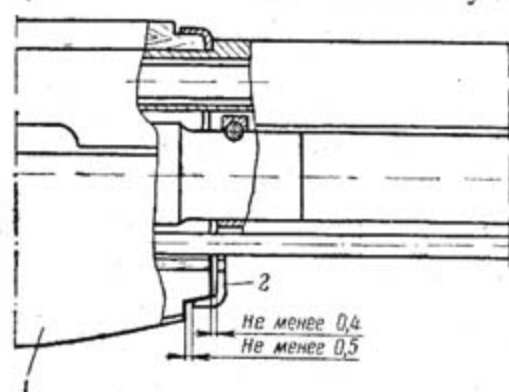
Рис. 71. Подгонка ложки к кольцу ложки: 1 — ложка; 2 — кольцо ложки
