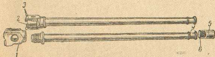
Рис. 2. Ствол.
