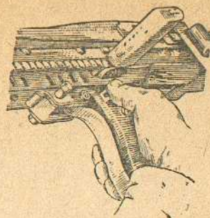
Рис. 16. Как поставить затвор на предохранитель
