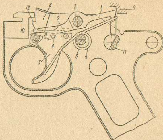
Рис. 23. Схема положения частей спускового механизма при затворе, находящемся на боевом взводе: 1 — шептало; 2 — ось шептала; 3 — спусковой крючок; 4 — ось спускового крючка; 5 — пружина; 6 — ось пружины; 7 — штифт; 8 — хомутик; 9 — боевой взвод затвора; 10 — рожки переднего конца шептала; 11 — предохранитель; 12 — выступы хомутика
