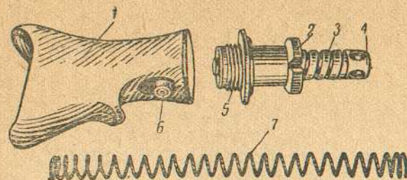
Рис. 9. Затыльник:
