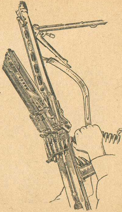
Рис. 17. Как зарядить пулемёт при питании из ленты
