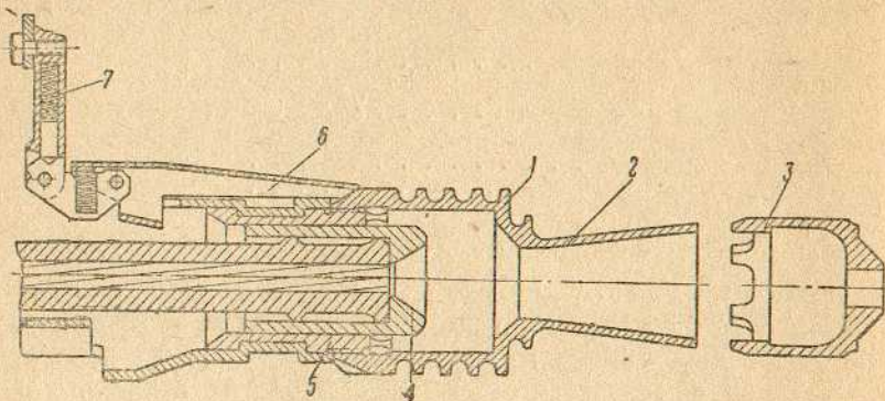
Рис. 3. Надульник:
