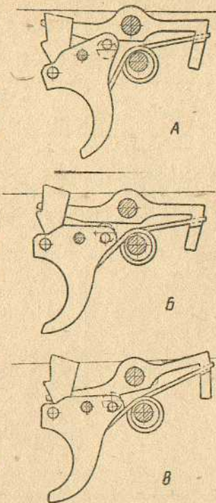
Рис. 24. Схема положения частей спускового механизма в различные периоды:
