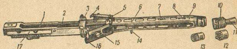
Рис. 5. Короб:
