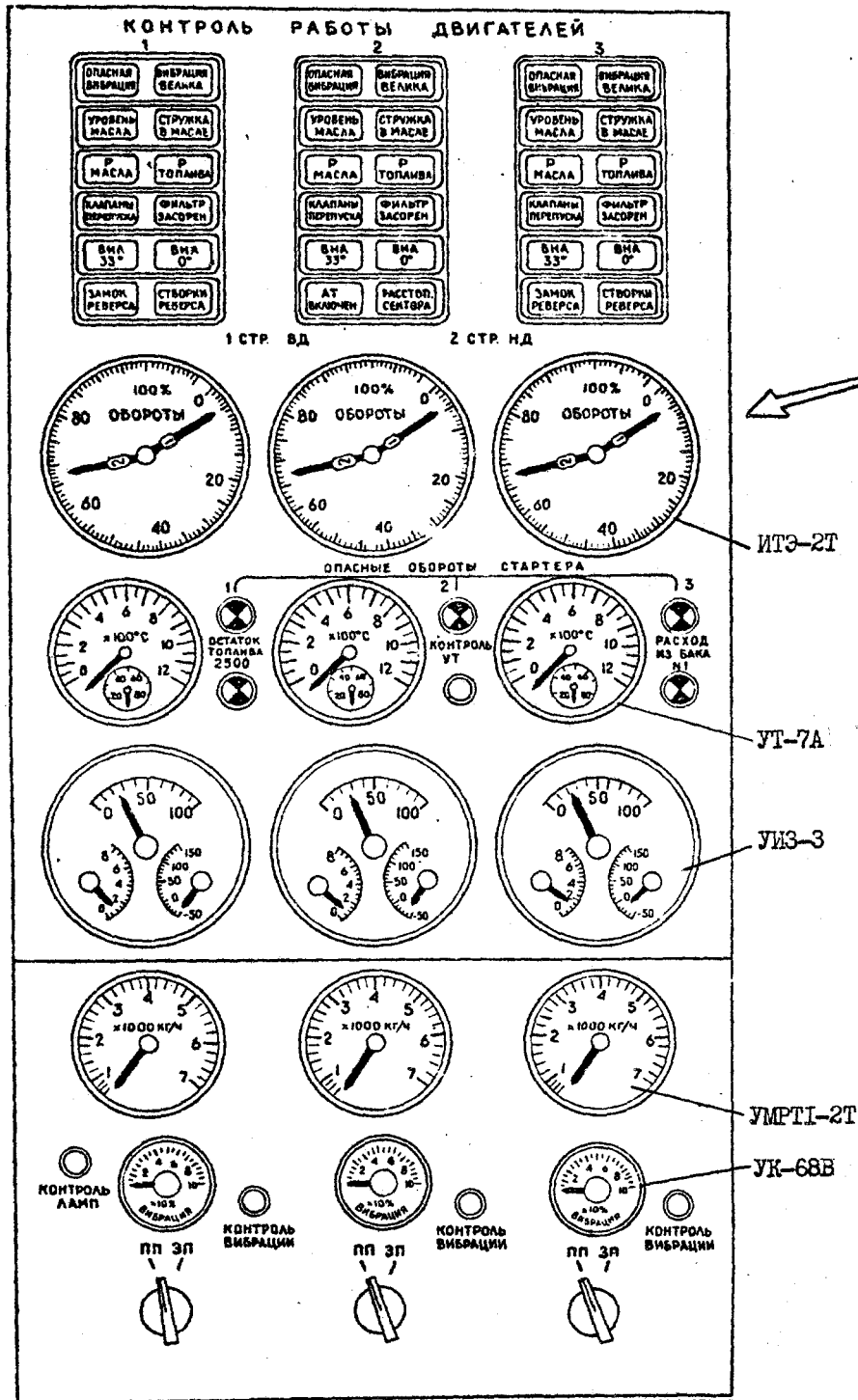
Панель приборов контроля двигателей на самолетах с № 818 * Рис. I (лист 2 из 2)
